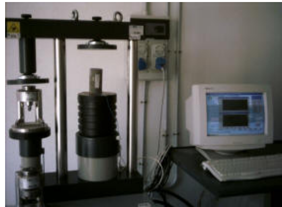
Determinazione del modulo elastico del calcestruzzo nel corso della prova di compressione
